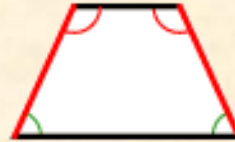
Isosceles trapezoid (Am.) Isosceles trapezium (Br.)
